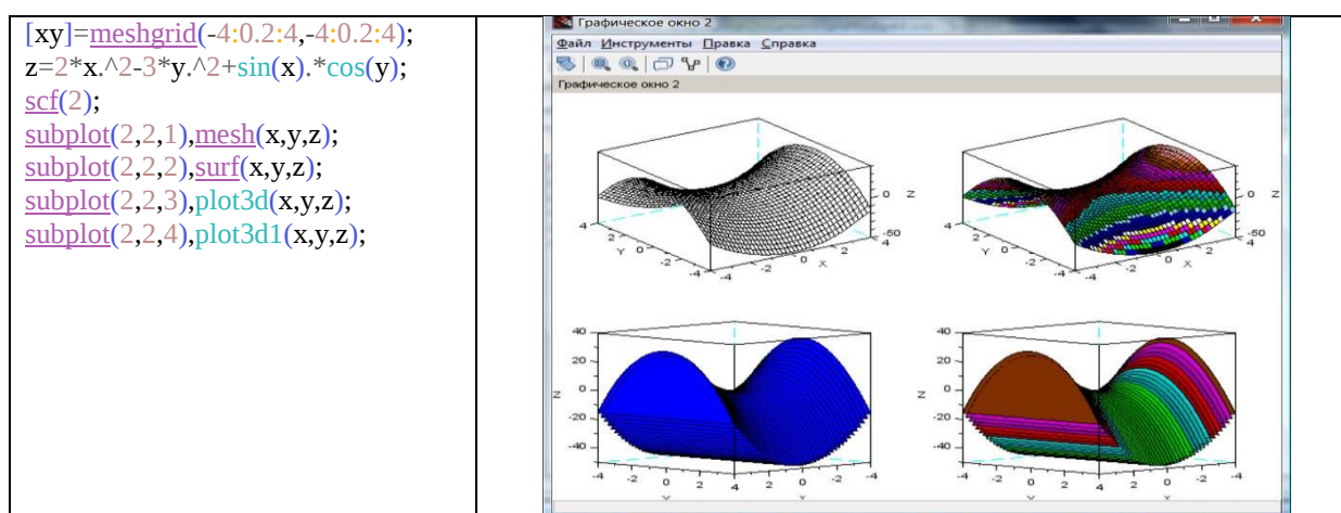
Рисунок 3 – Трехмерные графики функции, полученные с использованием различных команд в одном графическом окне
