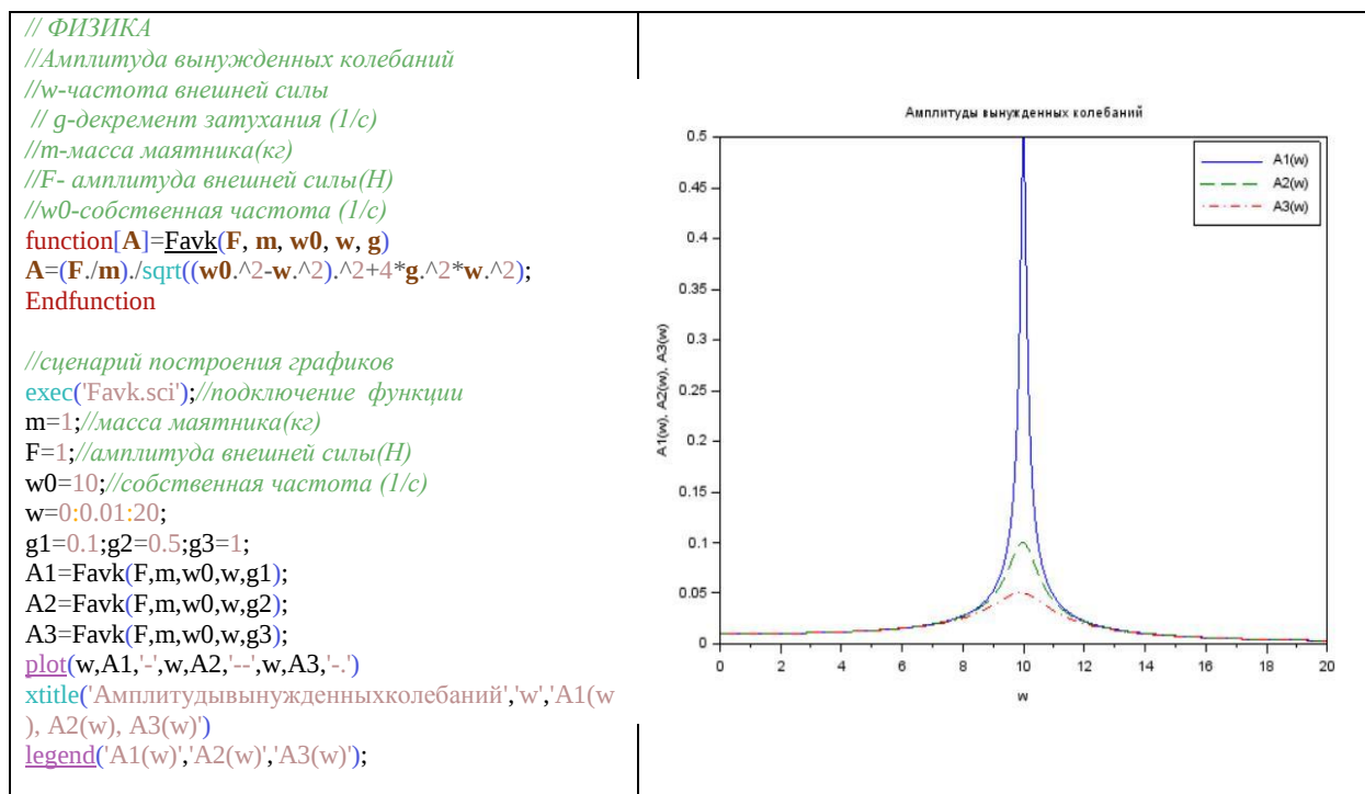
Рисунок 6 – Построение графиков амплитуды вынужденных колебаний
