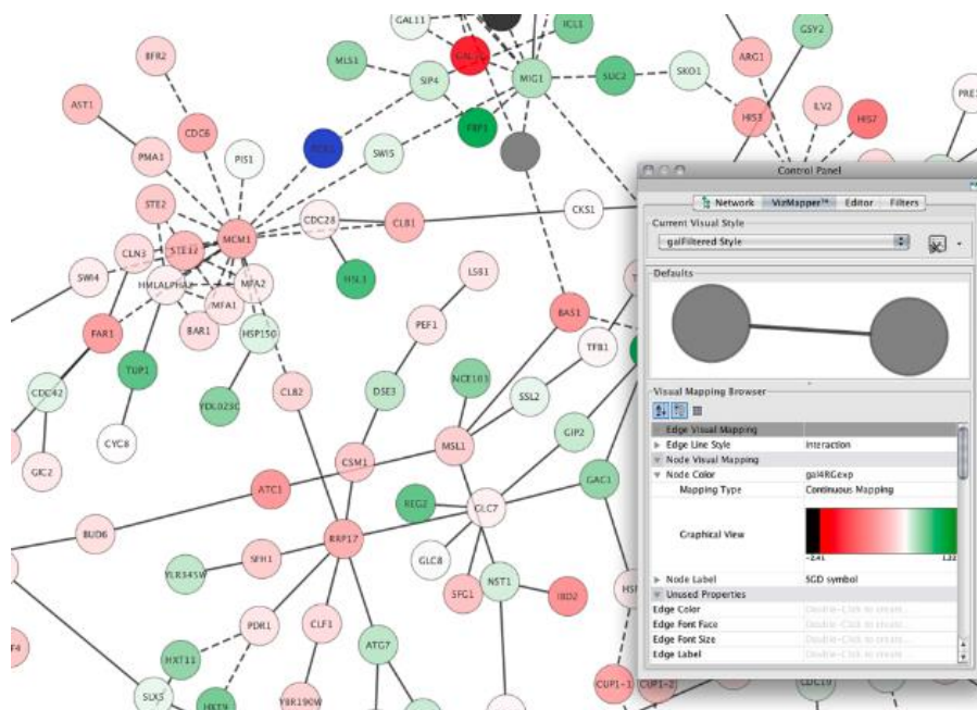
Рисунок 6 – Библиотека Cytoscape.js
