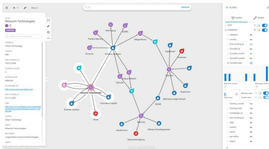
Рисунок 4 – Веб-платформа Linkurious
