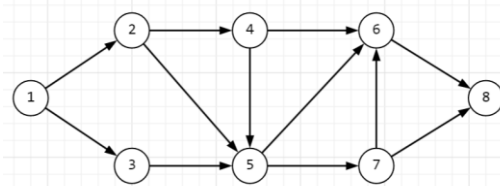
Рисунок 1 – Ориентированный граф
